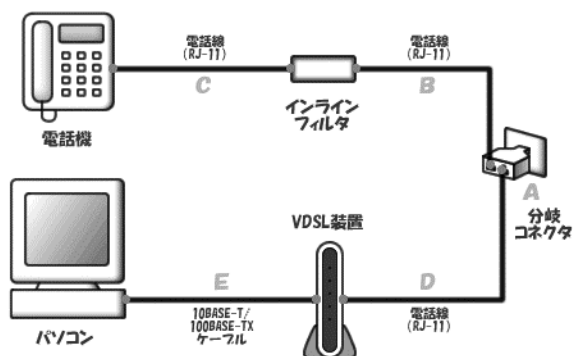
図1 宅内の VDSL の基本構成
