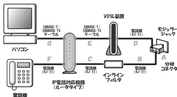
b. IP 電話機対応機器(ルータタイプ)の使用
