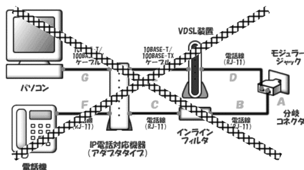
a. IP 電話機対応機器(アダプタタイプ)の使用
